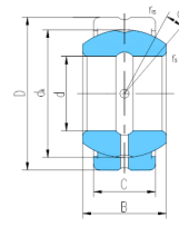
GEZ...ES-2RS
