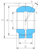
GEZ...ES
